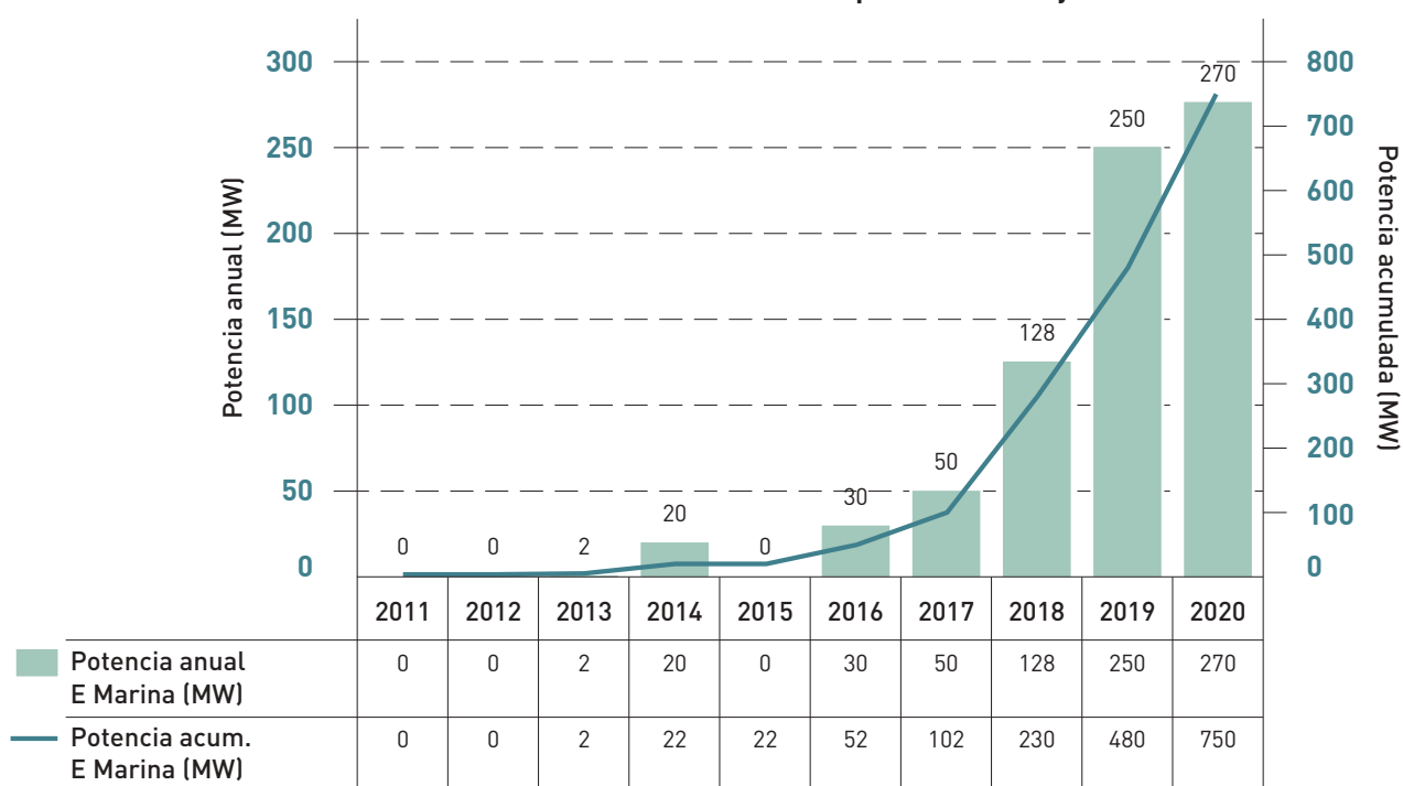
Figura 4.5.17. Previsiones de potencia eólica marina anual en España, horizonte 2020
