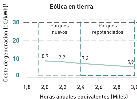
Figura 4.5.8. Sensibilidad de los costes normalizados de energía de un parque eólico en tierra a la producción
