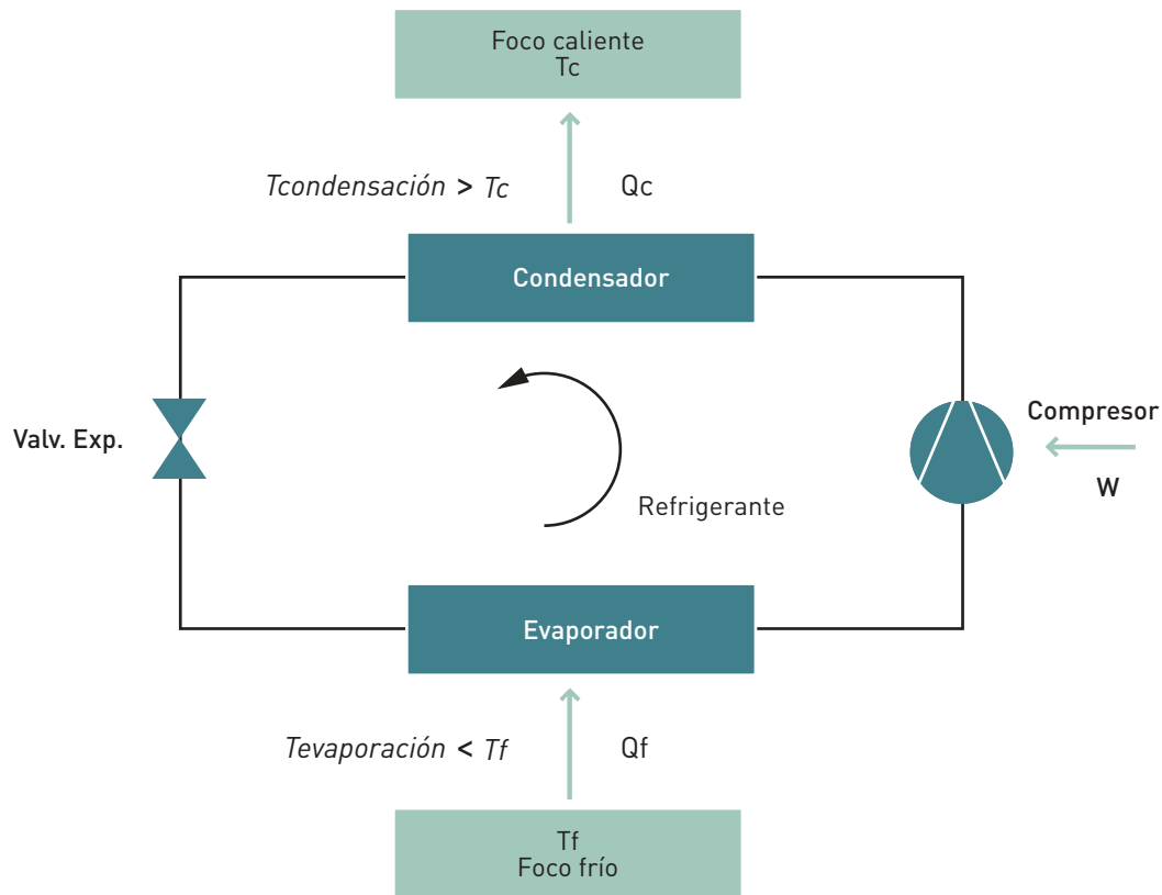
Figura 4.6.19. Esquema básico de una bomba de calor
