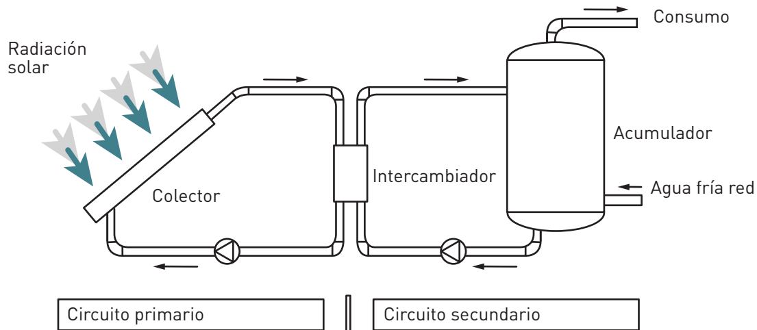
Figura 4.10.9. Esquema típico de instalación solar térmica para ACS
