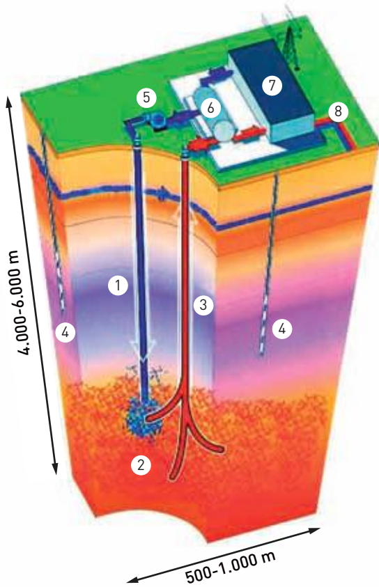
Figura 4.6.16. Esquema simplificado de un aprovechamiento de roca caliente seca o sistema geotérmico estimulado
