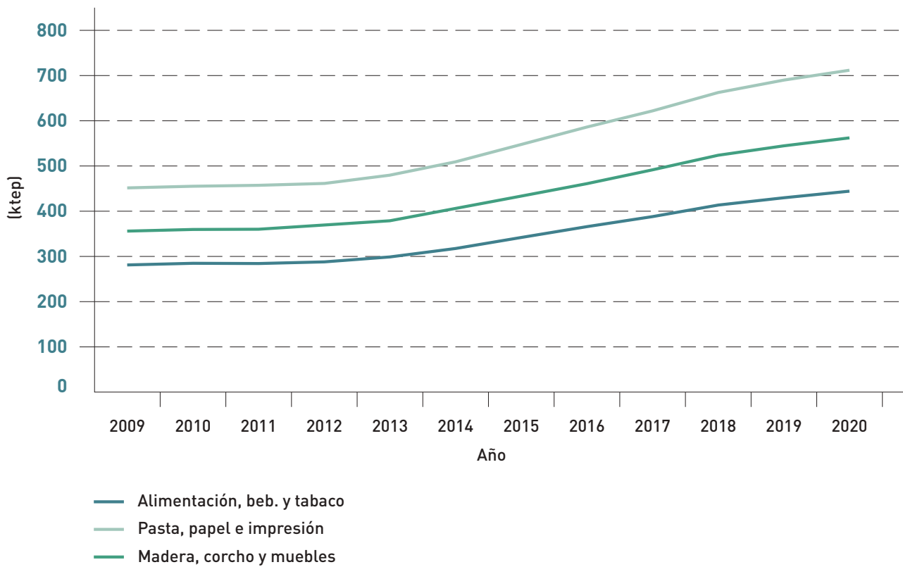
Figura 4.3.16. Consumo térmico por subsectores
