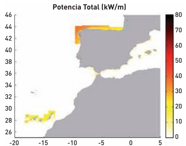
Figura 4.4.16. Atlas de potencia media del oleaje en España (kW/m)
