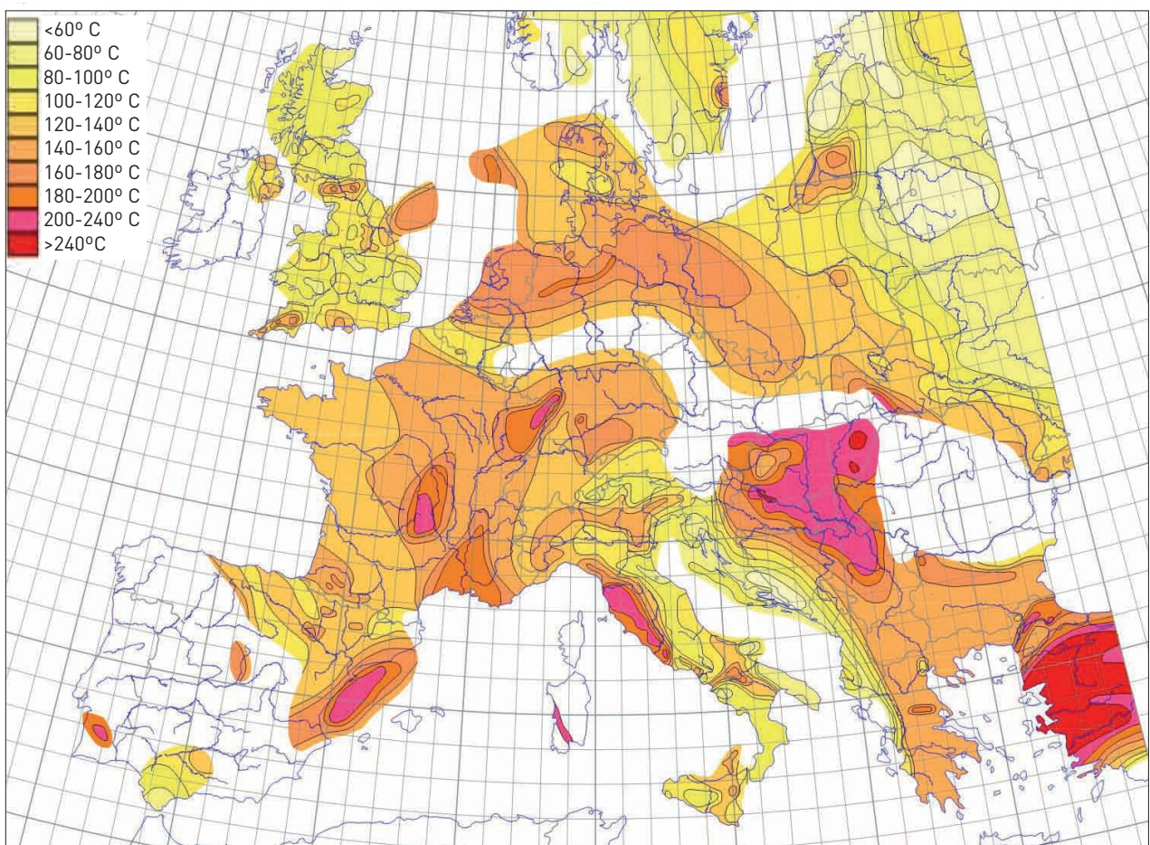
Figura 4.6.5. Extrapolación de temperaturas a 5 km de profundidad
