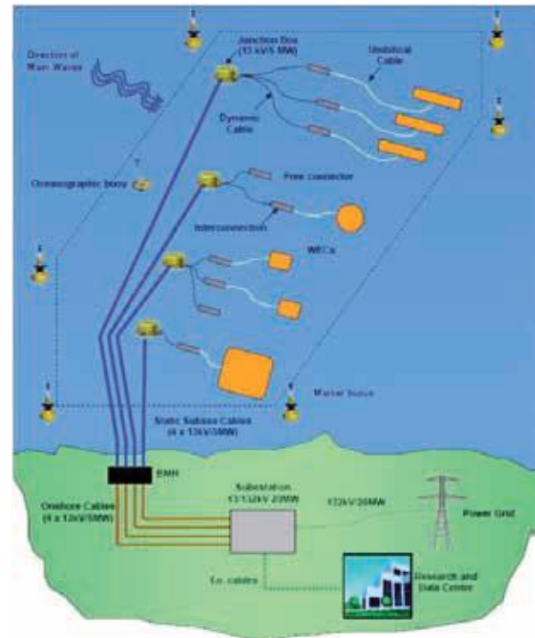
Figura 4.4.13. Arquitectura conceptual de la infraestructura de BIMEP
