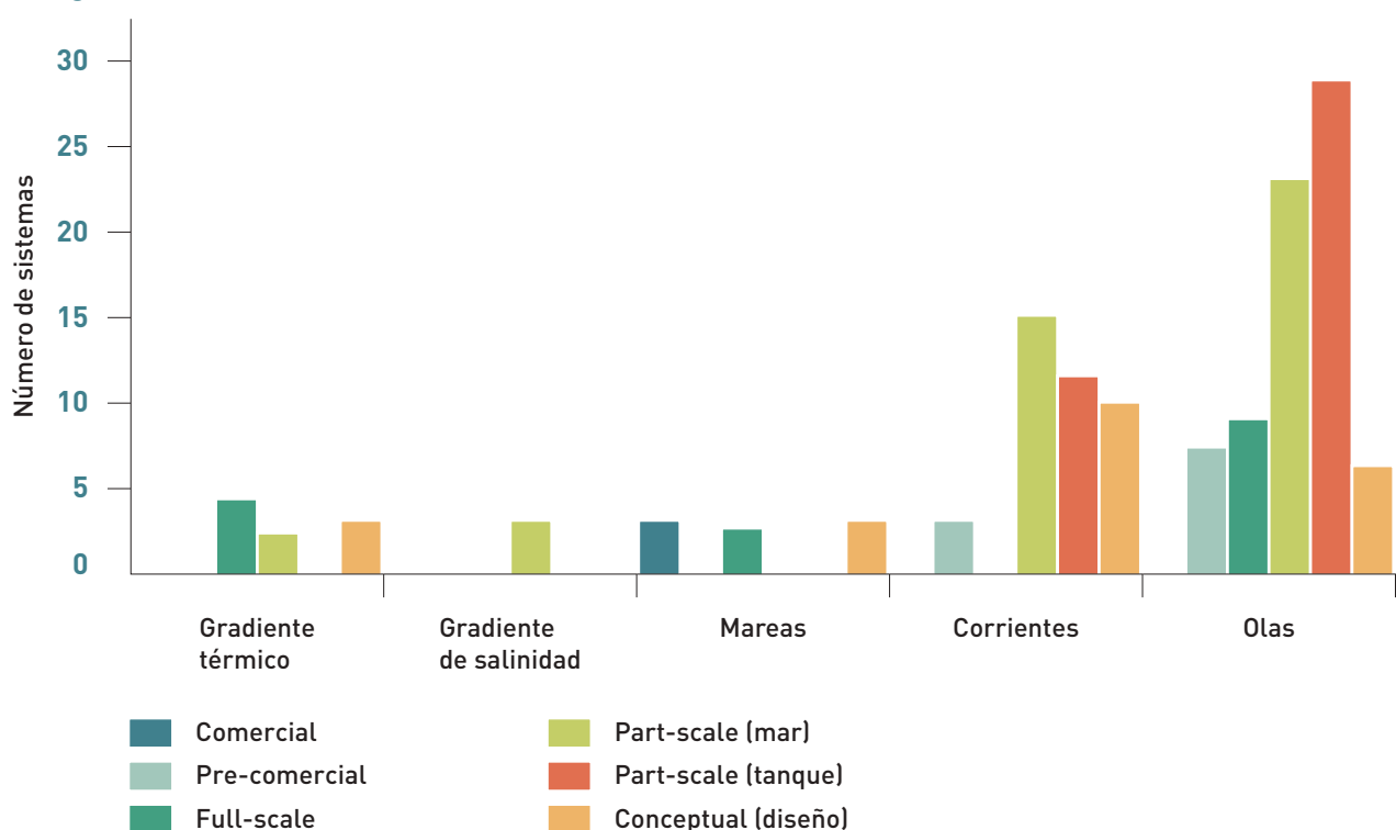
Figura 4.4.8. Estado de desarrollo y madurez de las distintas tecnologías de aprovechamiento de energías del mar
